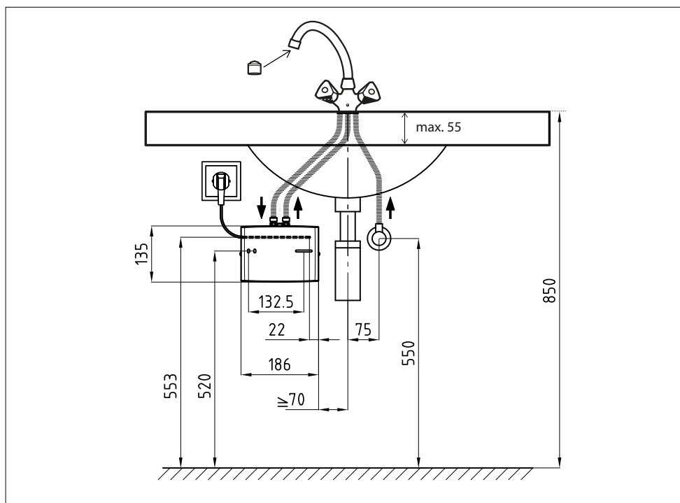
Abb. 3: »Installation mit Armatur« (Maßangaben in mm)
