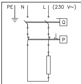
Abb. 6: »Schaltplan«
