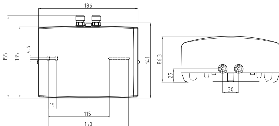
Abb. 1: »Abmessungen« (Maßangaben in mm)
